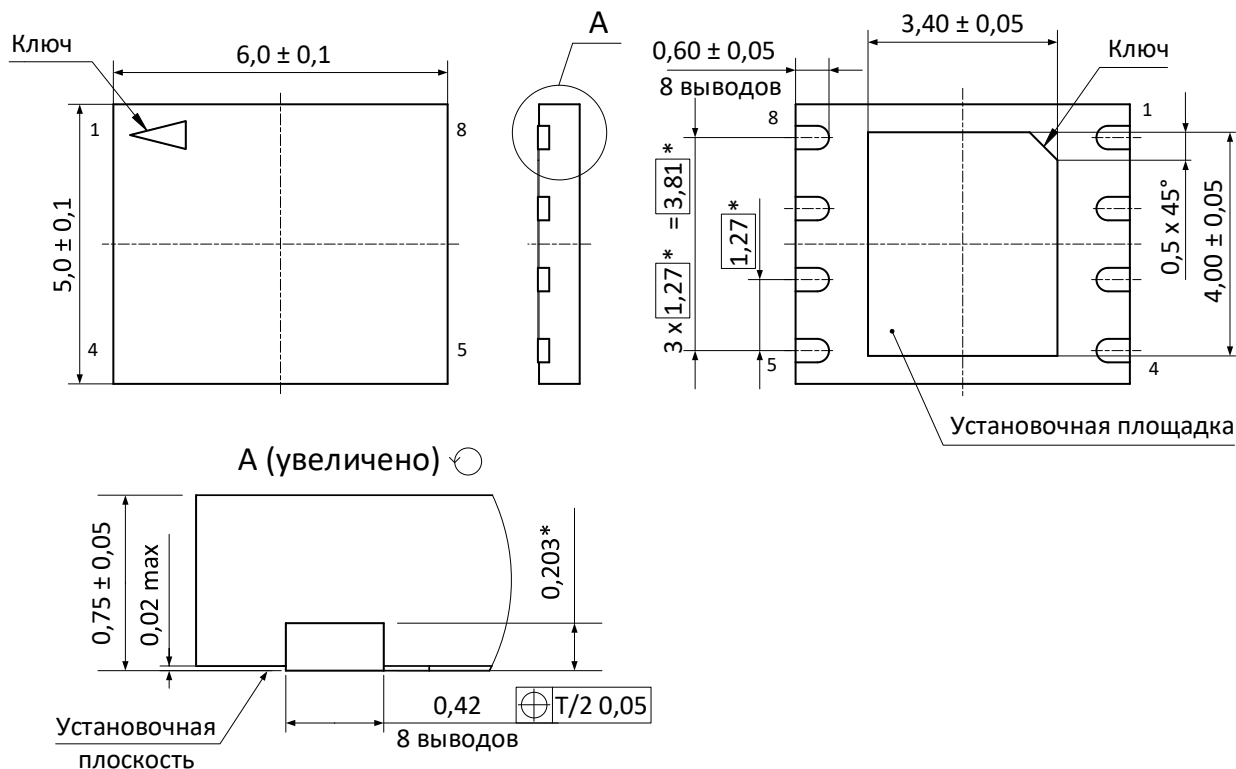
Рисунок 11 – Микросхема в корпусе DFN8 5×6×0,75 (1,27)
